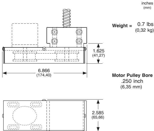
NEMA 23 Right Hand Motor Wrap (M06)
