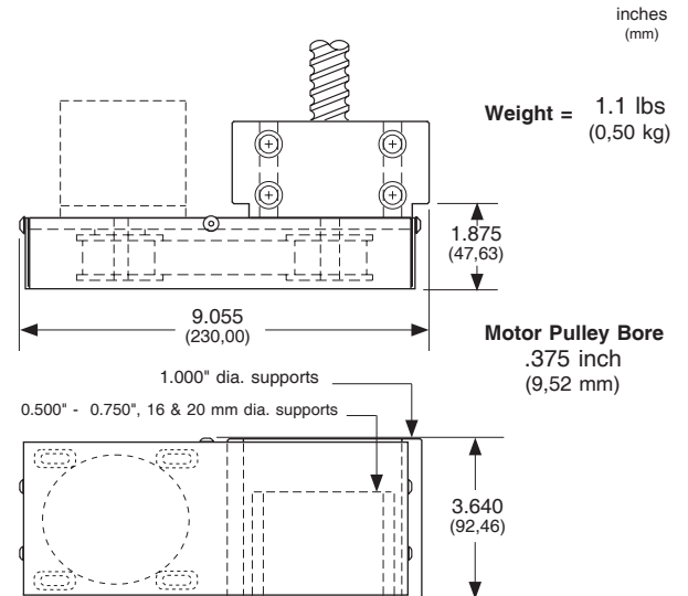
NEMA 34 Right Hand Motor Wrap (M08)
